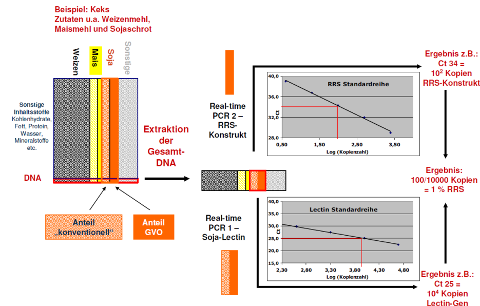
Abb. 4: Prinzip der Quantifizierung gentechnischer Veränderungen mittels Real-time PCR am Beispiel von Roundup Ready® Soja (RRS). Nach Extraktion der DNA des Lebensmittels wird diese in 2 parallelen real-time PCR Reaktionen untersucht. In Real-time PCR 1 wird als Referenz die Menge (als Genomäquivalente = Kopien) der spezies-spezifischen Soja-Lectin-Gensequenz, in real-time PCR 2 die Menge einer Sequenz aus dem für RRS spezifischen Konstrukts bestimmt. Für die Quantifizierung der Lectin bzw. RRS-Kopienzahl wird davon ausgegangen, dass in einem 100 % RRS-Standard die Lectin- und die RRS-spezifische Sequenz im Verhältnis 1:1 und jeweils als „single-copy“-Sequenzen einmal in jedem Genom vorkommen. Die Quantifizierung kann dann mittels DNA aus Referenz-Standards (z.B. Mehlen) erfolgen, die einen definierten Anteil an RRS aufweisen (z.B. 5 % RRS w/w). Die Referenz-DNA wird in verschiedenen Verdünnungsstufen, entsprechend einer Standardreihe für die Lectin- und die RRS-Sequenz untersucht. Die für die Proben-DNA jeweils erhaltenen Ct-Werte oder Crossing points werden über die jeweiligen Regressionsgeraden (Ct gegen logKopienzahl) Kopienzahlen zugeordnet. Die Kopienzahlen für die RRS- und die Lectin-Sequenz werden zueinander ins Verhältnis gesetzt. [11, 29].
