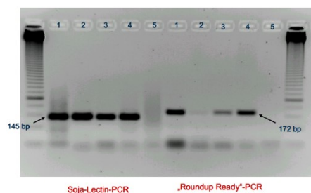
Abb. 2: Qualitative (=Endpunkt)-PCR zum Nachweis gentechnisch veränderter Soja in Sojalecithin [19]. Agarosegel-Elektrophorese nach Amplifikation eines 145 bp Abschnitts des Soja-Lectin-Gens (Amplifikationskontrolle der extrahierten DNA) (links) bzw. einer für das Roundup-Ready®-Soja (RRS)-Konstrukt spezifischen Sequenz (172 bp) (rechts).
