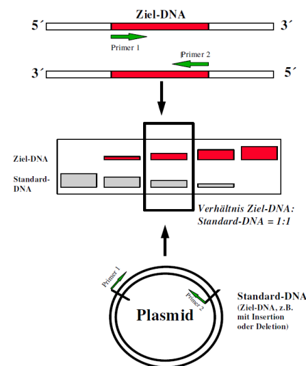
Abb. 3: Prinzip der kompetitiven PCR.
