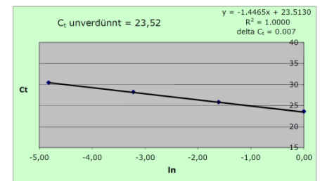
Abb. 1: Überprüfung der DNA-Extraktion auf Inhibition mittels Verdünnungsreihe [21]. Verdünnungsreihe eines DNA-Extraktes aus Sojalecithin (1+4, 1+24 and 1+124). Ct-Werte aus der Amplifikation einer Soja-Lectin-Gen-Sequenz mittels Real-time PCR (y-Achse) sind gegen den natürlichen Logarithmus (ln) des jeweiligen Verdünnungsfaktors aufgetragen (0,2, 0,04 bzw. 0,008). Der über Extrapolation der Geraden zur y-Achse erhaltene Ct-Wert wird mit dem Messwert der unverdünnten DNA verglichen (delta Ct).
